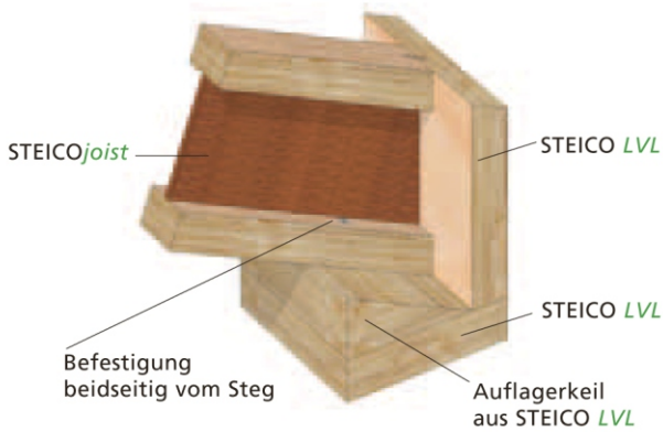
D5 Traufe mit Auflagerkeil
