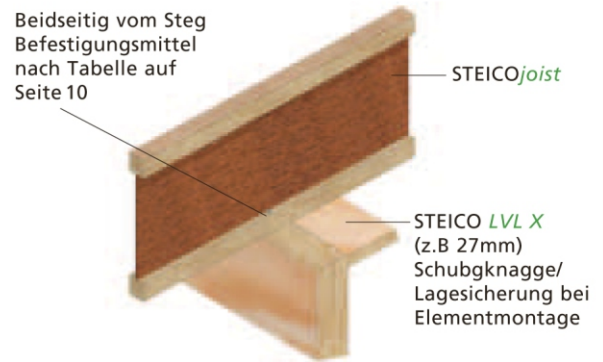
D4 Mittelpfettenanschluss mit STEICO LVL X Schubknagge
