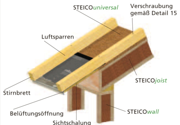
D8 Traufe mit Luftsparren nicht sichtbar
