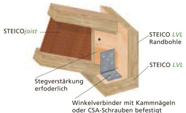
D6 Waagrechtes Auflager
